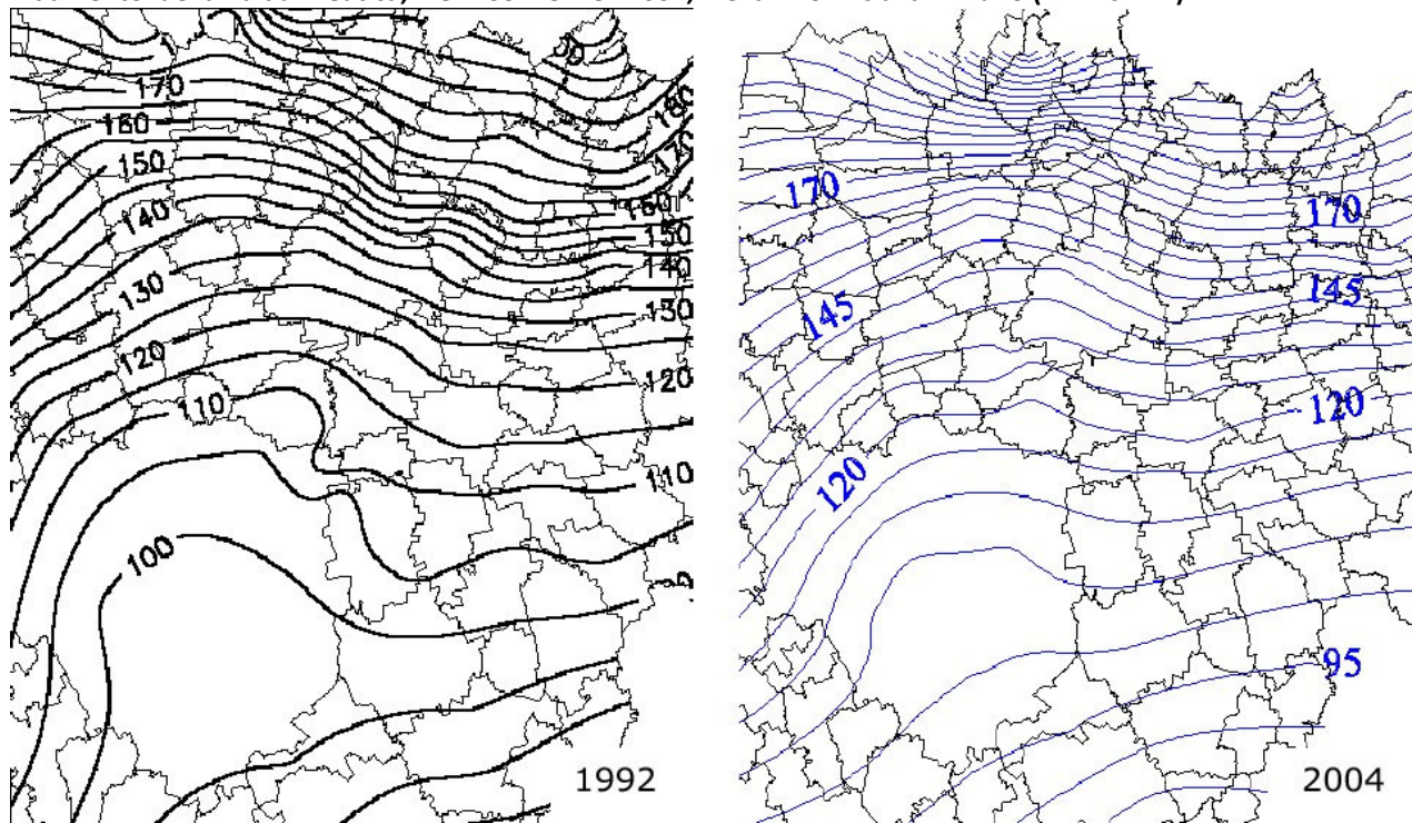
Andamento della falda freatica, nel 1992 e nel 2004, nella Provincia di Milano (in m s.l.m.)
